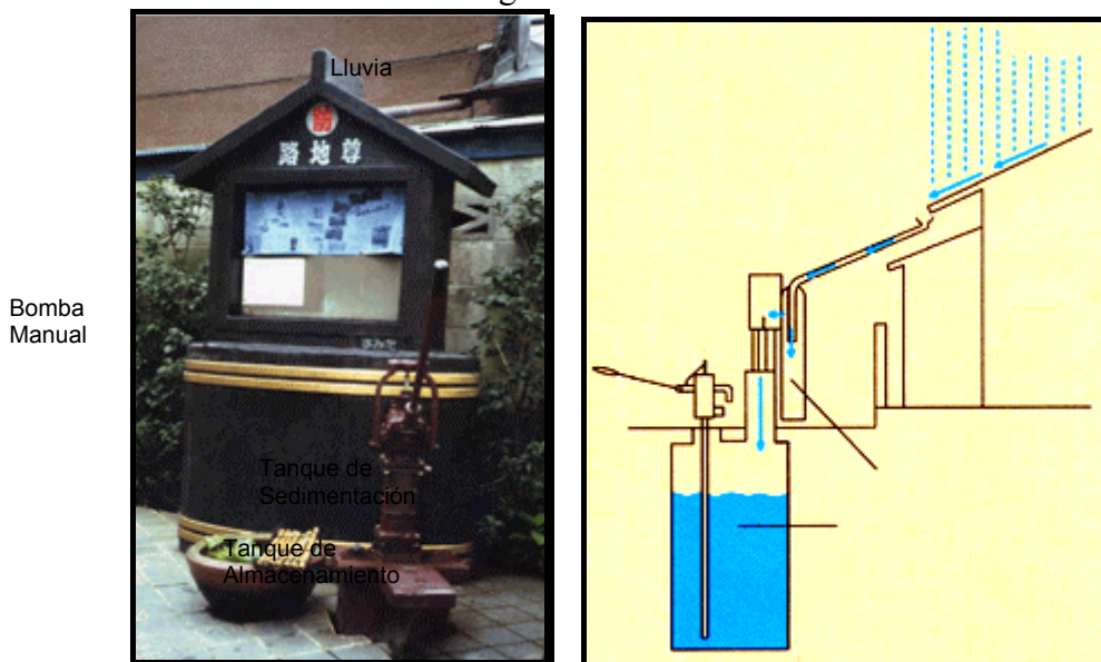
Figura N° 2. “Rojinson”, instalación para la utilización de agua lluvia a nivel comunitario en Tokio, Japón.
